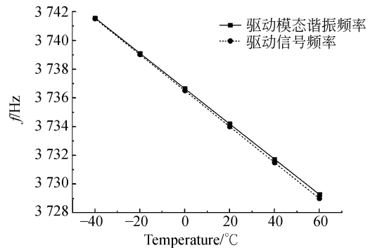
图 4 驱动信号频率与驱动模式谐振频率随温度变化曲线
