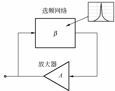
图 1 自激振荡基本原理图 [9]
