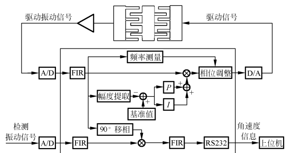
图 2 FPGA 数字控制系统结构图
