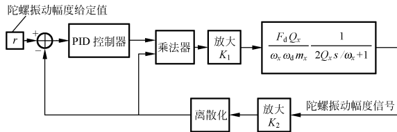
图 3 自激驱动电路幅度控制原理图
