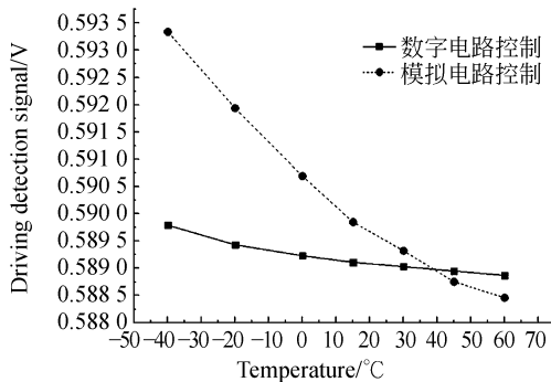
图6 数字和模拟方式控制的幅度随温度变化曲线
