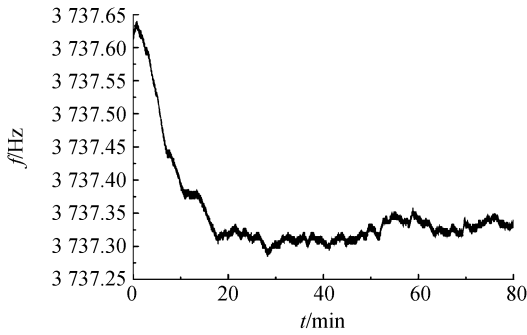
图5 从启动到80 min陀螺驱动信号频率漂移曲线
