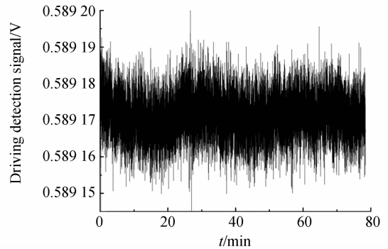
图7 从启动到80 min陀螺驱动信号幅度漂移曲线
